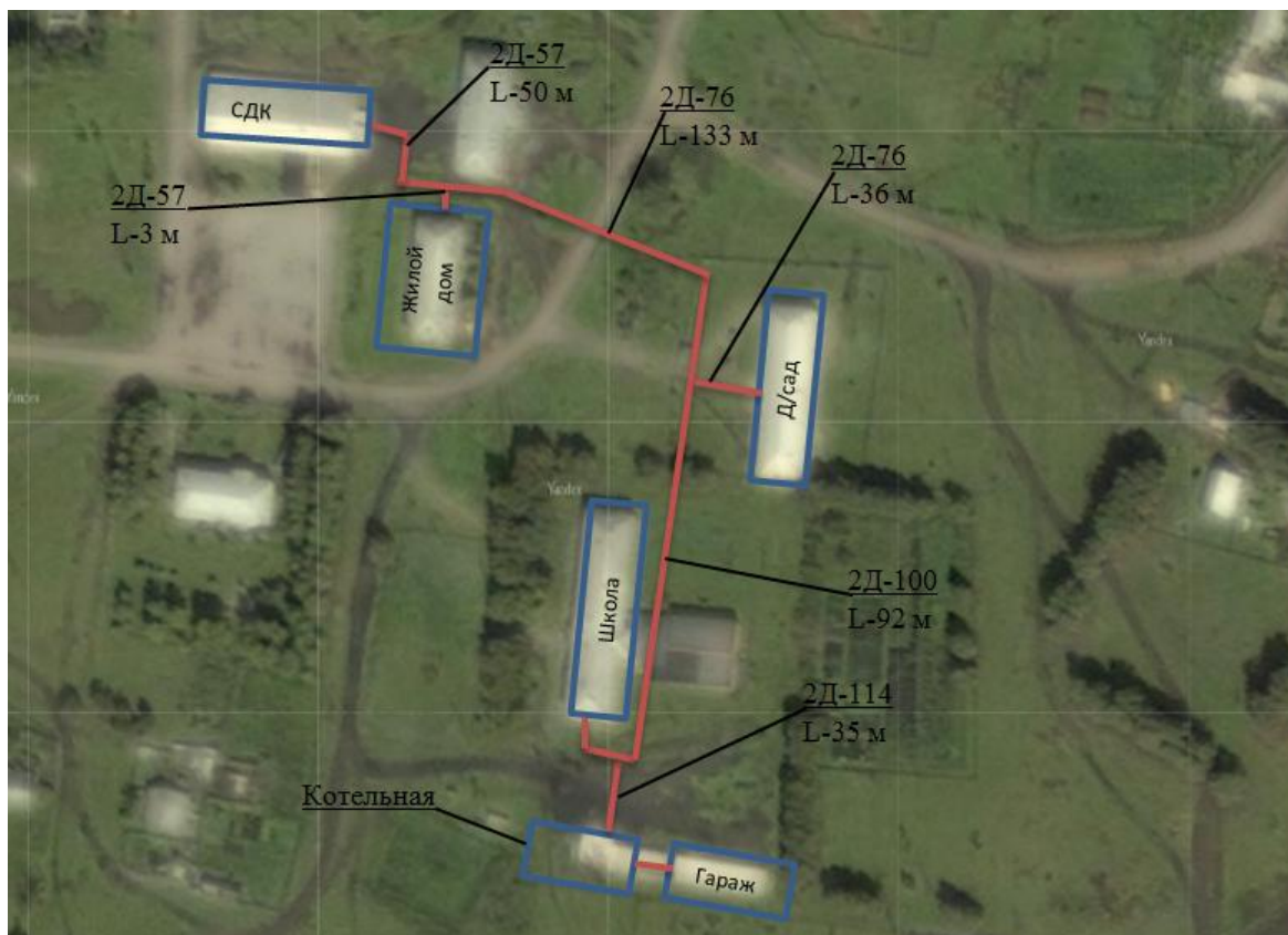
Рис. 2. Существующая зона действия котельной СОШ с. Троицкое
